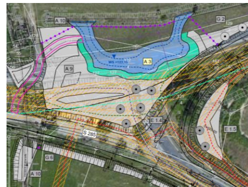
Ausschnitt Ausführungs Lageplan zur Maßnahme A 3
