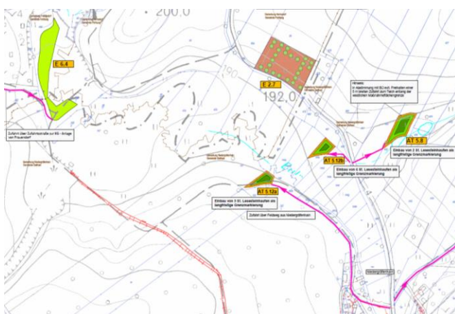
Ausschnitt Ausführungsanlageplan, Eulaaue zwischen Niedergräfenhain und Hermsdorf: Maßnahmen AT 5.8, AT 5.12, E 2.7 und E 6.4
